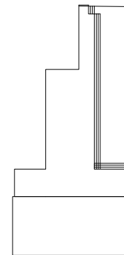
날개벽(우측)
